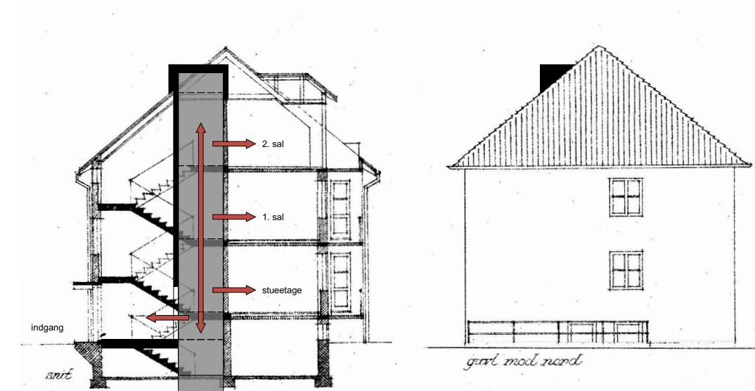
Principsnit gennem elevatorskaft med 1m overhøjde og grube
