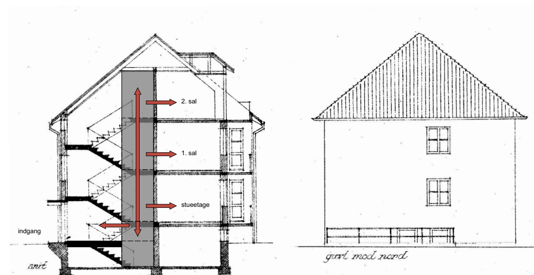
Principsnit gennem elevatorkift uden overhøjde og grube
